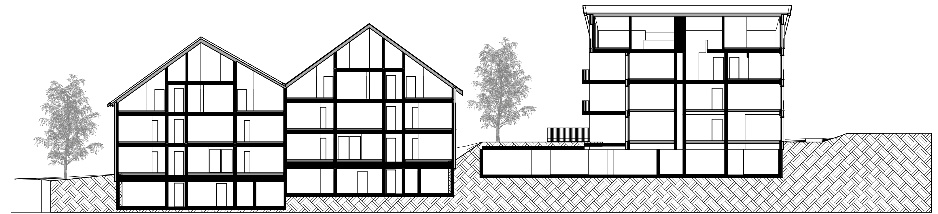
Schnitt A-A
