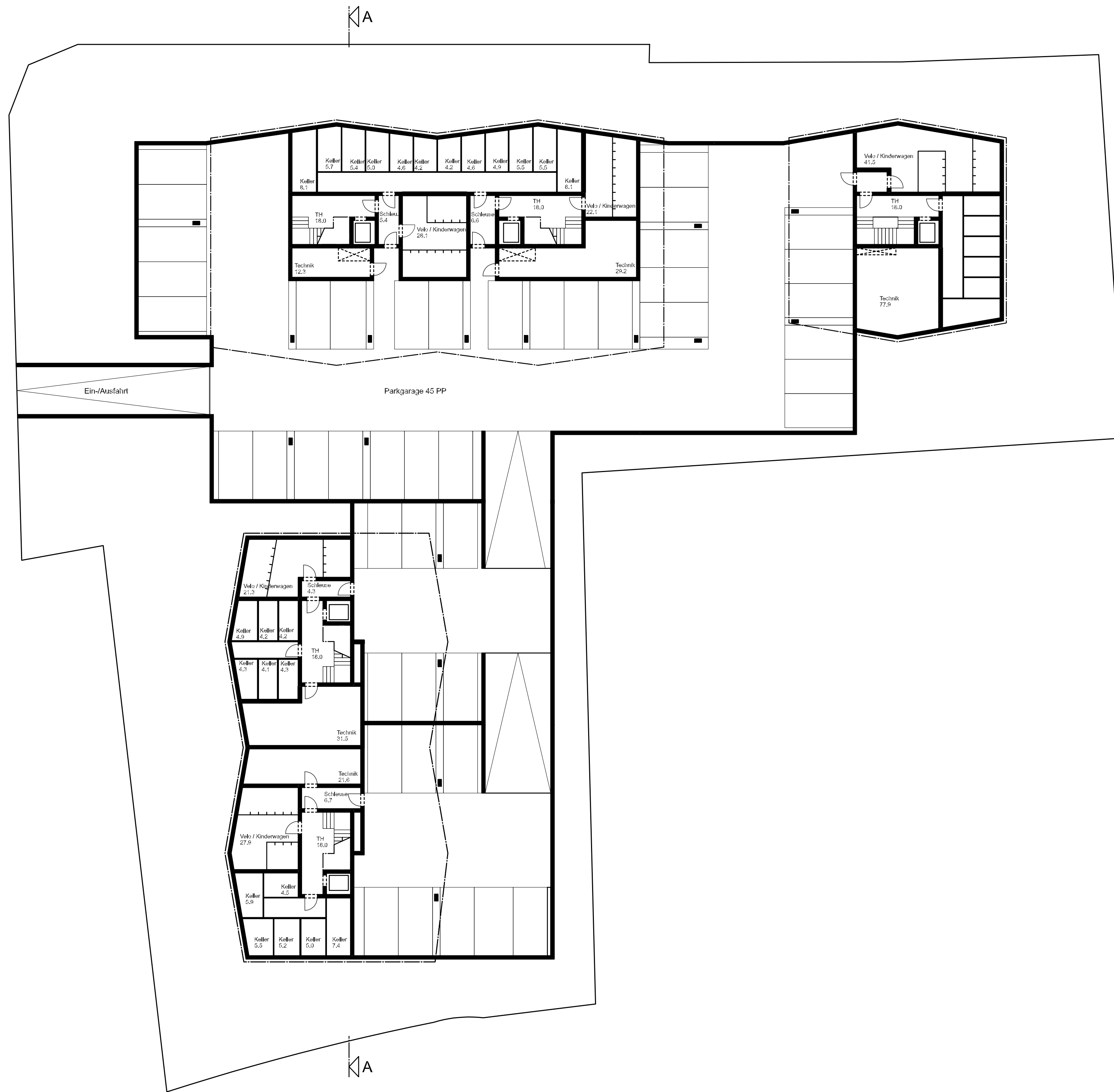
Untergeschoss
