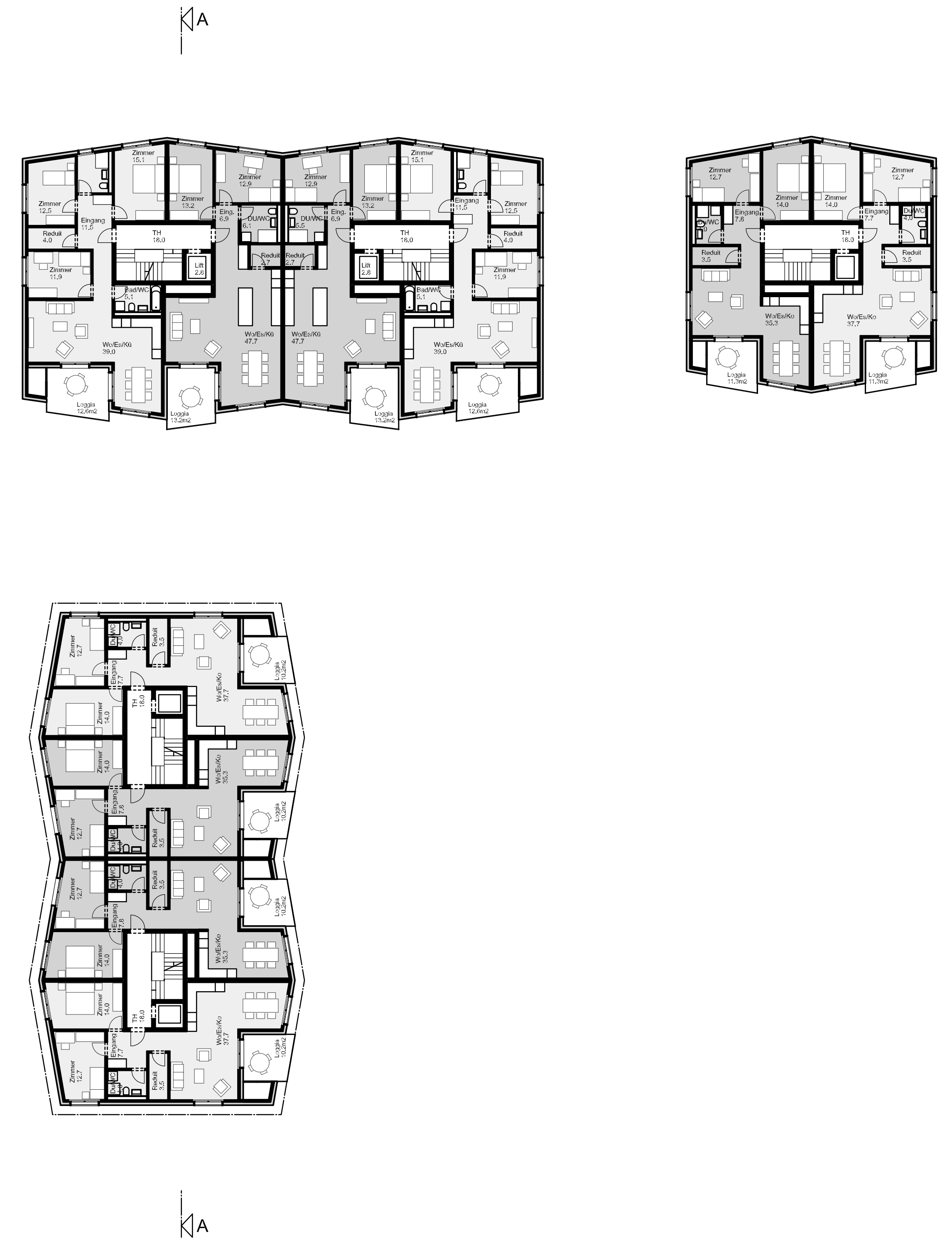
Obergeschoss
